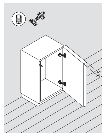
25mm厚度的门板 (带弹簧铰链, 有无阻尼均可)
