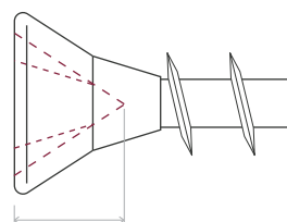
增加十字槽深度上限
